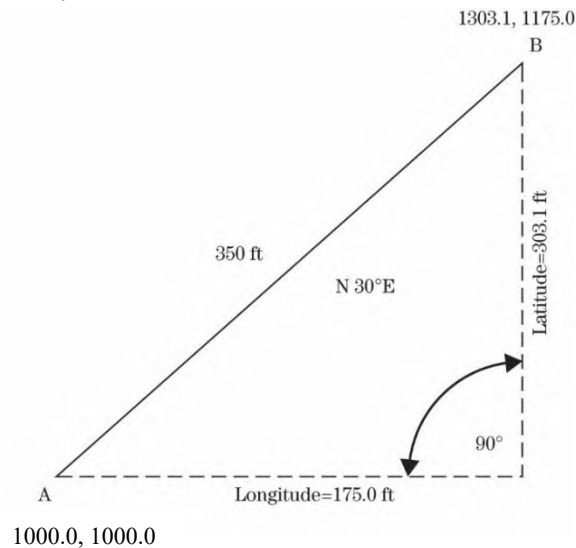
Figure 1-17: Calculating Horizontal Latitude and Longitude Coordinates from Survey Data
