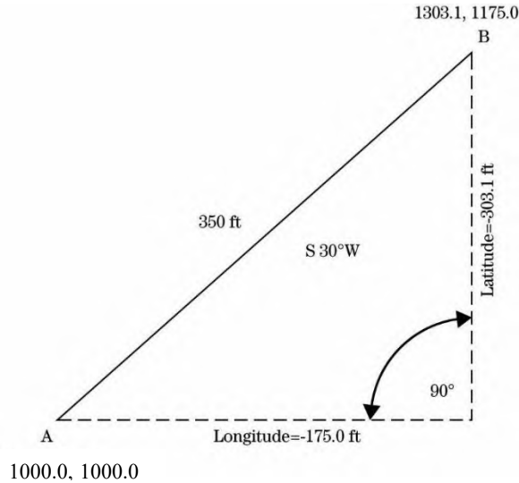
Figure 1-18: Calculating Horizontal Latitude and Longitude Coordinates from Survey Data
